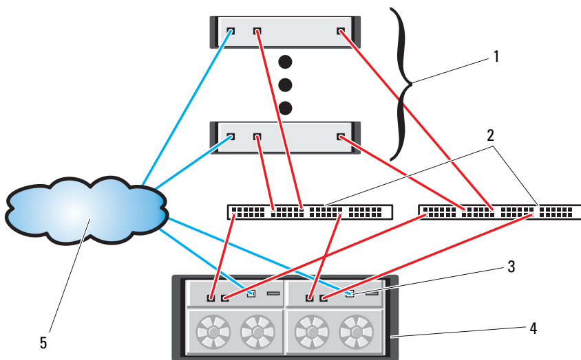
図 1-6. iSCSI スwitch 式クラスタのケーブル接続
